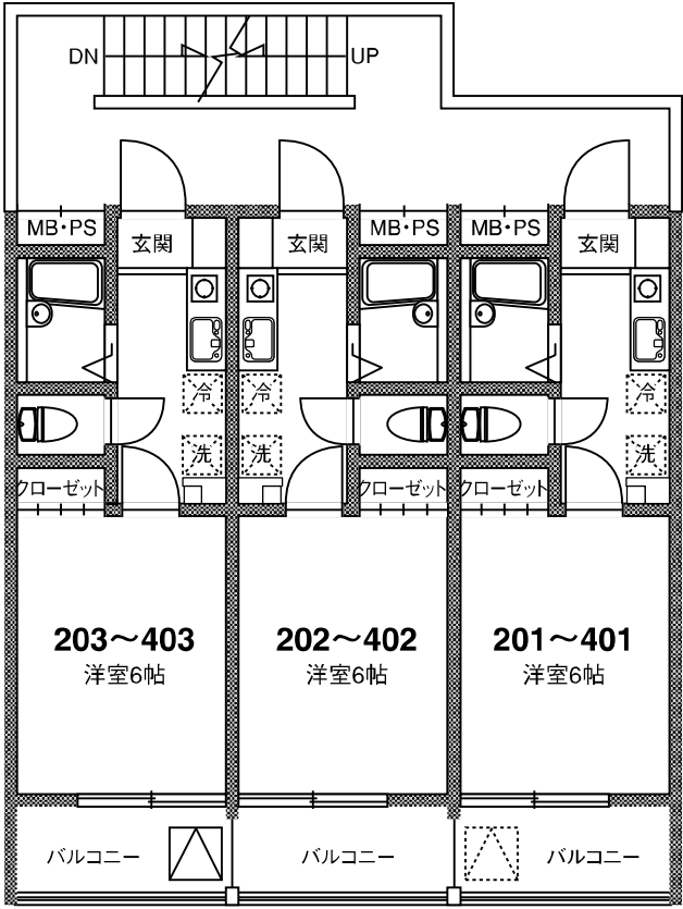
2-4階 平面図
