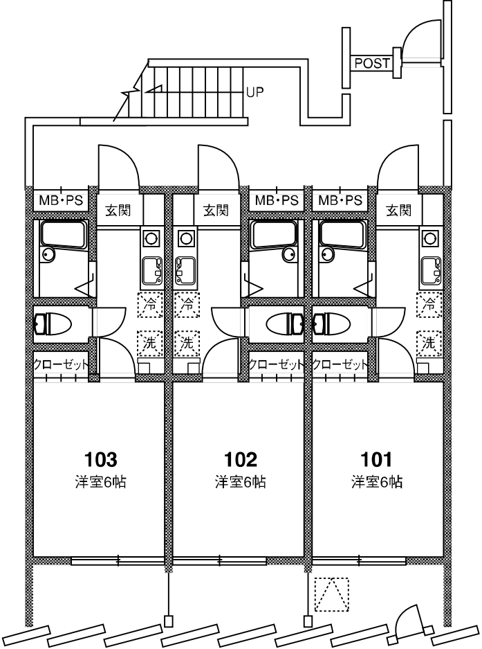
1階 平面図
